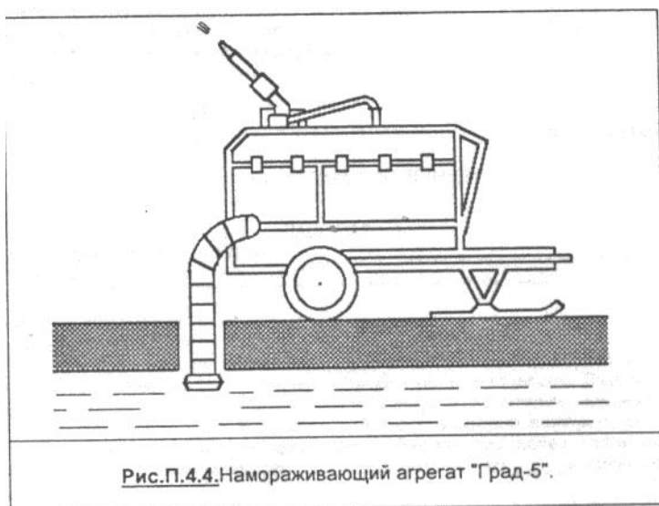
Рис. П.4.4. Намораживающий агрегат "Град-5"
