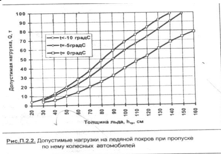
Рис. П.2.2. Допустимые нагрузки на ледяной покров при пропуске по нему колесных автомобилей
