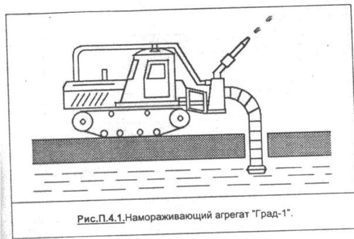
Рис. П.4.1. Намораживающий агрегат "Град-1"
