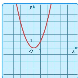
Рис. 1. График функции y(x) = x^2
